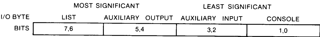
Figure 4-3. I/O Byte
